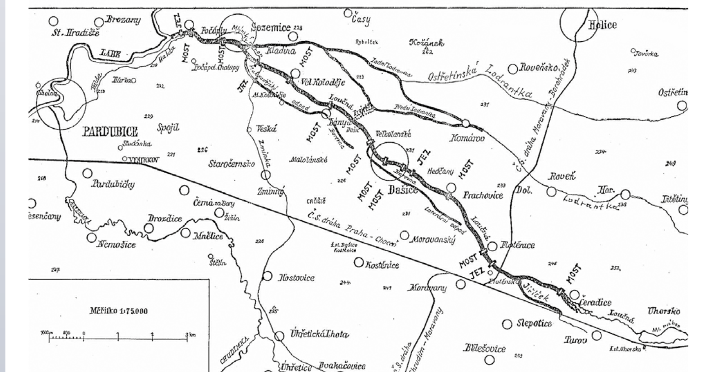
Situace provedených úprav Vodním družstvem pro úpravu řeky Loučné a potoka Lodrantky v Dašicích, okres Pardubice.
